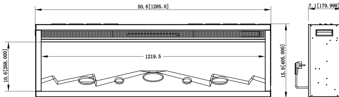
Rysunek techniczny
